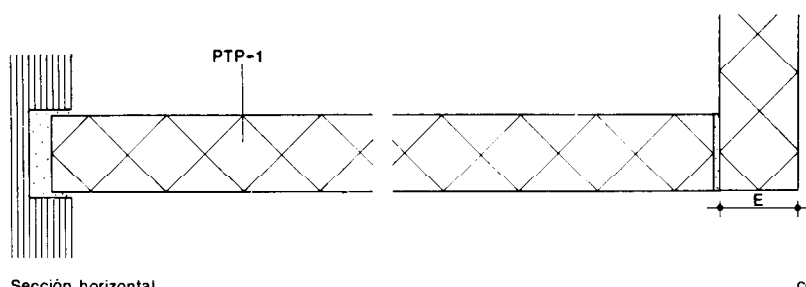
Sección horizontal
