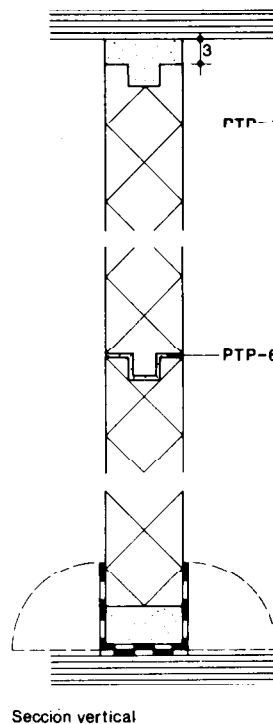
Sección vertical
