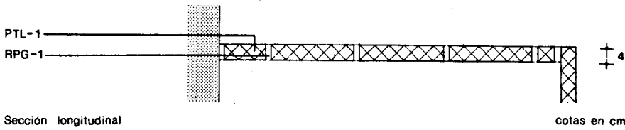
Sección longitudinal
