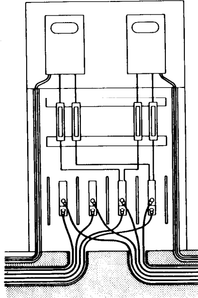
Sección
