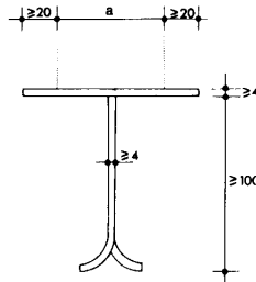
Alzado
