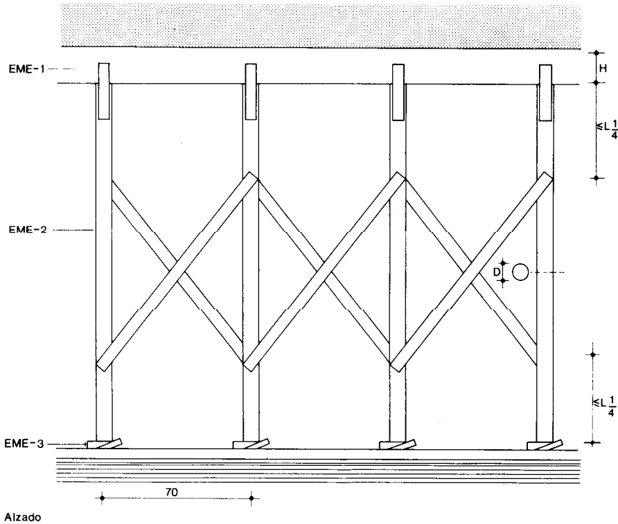
Alzado
