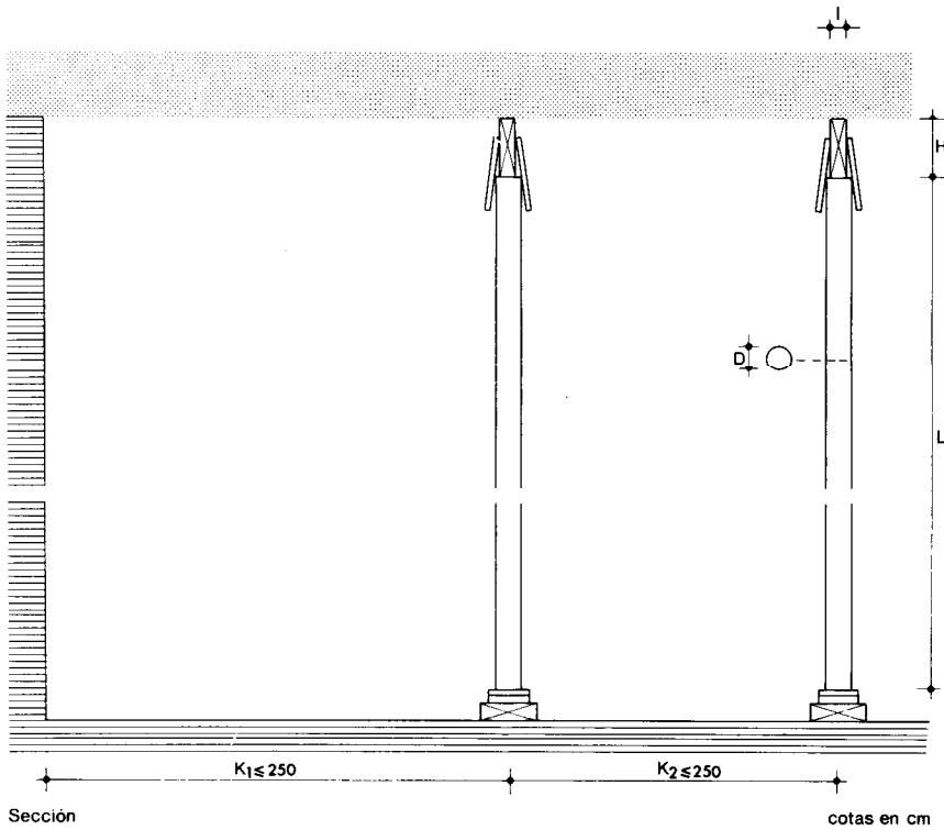
Sección
