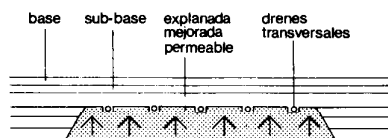
Sección A-A
