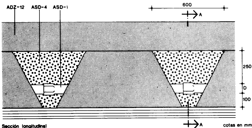
Sección longitudinal
