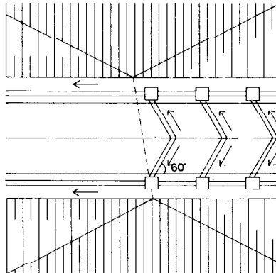
Planta Paso de desmorte a terraplén
