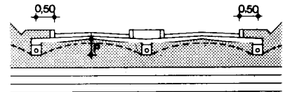
Calzada doble
