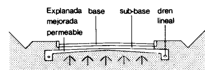
Drenaje de agua ascendente Sección transversal
