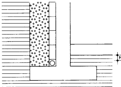
Sección vertical
